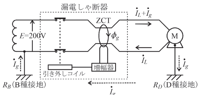
図 6.3 等価回路
