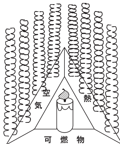
図 3.1 火の三角形
