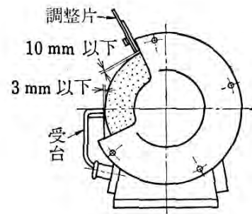
図 4.8 受台・調整片の隙間
