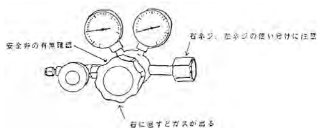
図 9.2 圧力調整器
