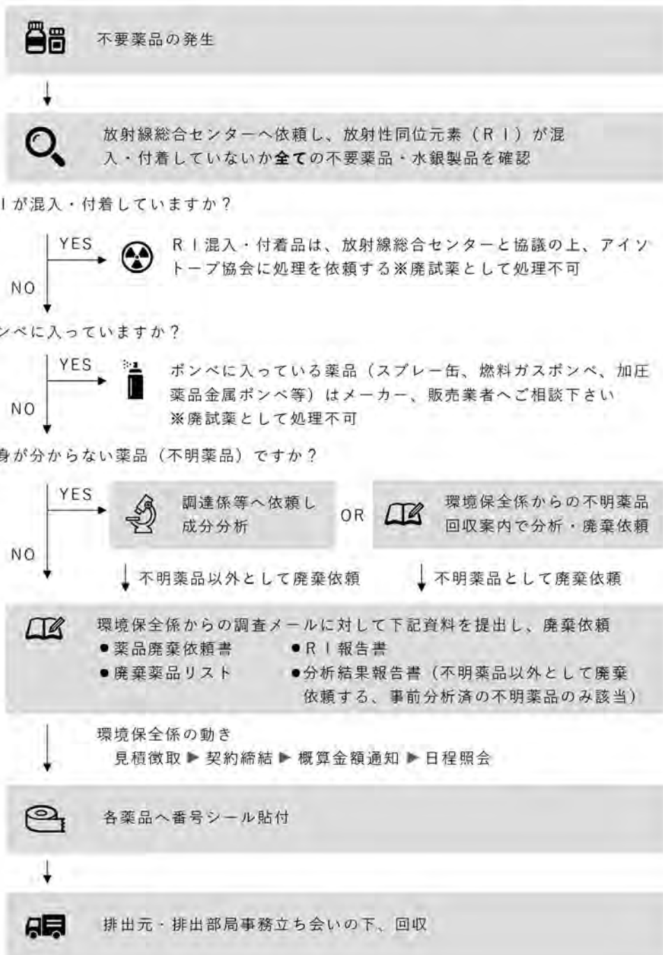
図 13.5 廃棄試薬処理の手順
