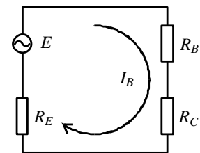
図 6.2 等価回路
