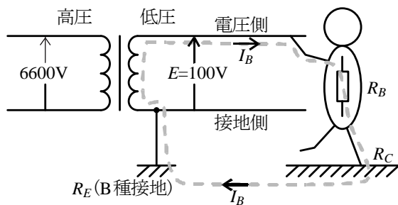
図 6.1 感電発生メカニズム
