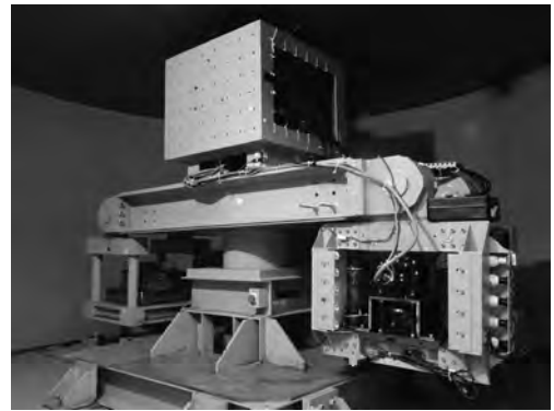
図 7.3 遠心载荷装置
