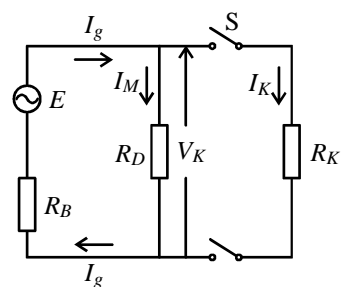
図 6.5 等価回路
