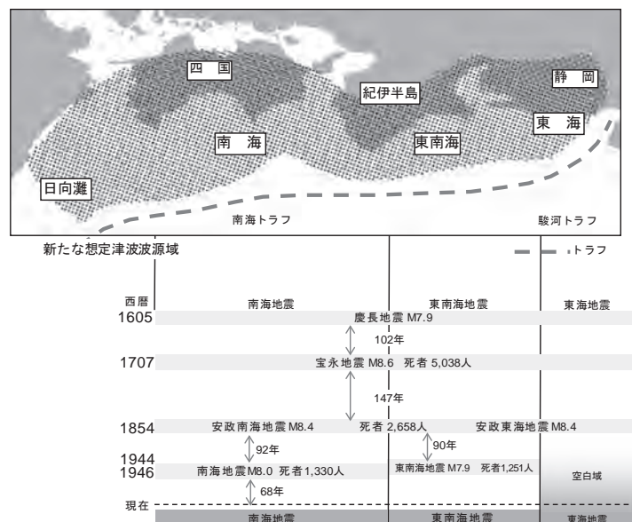
図 3.2 南海トラフ地震の発生状況 (1600 年以降)
