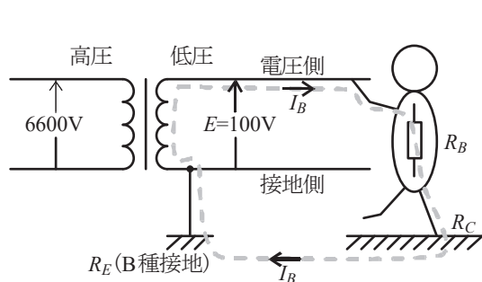
図 6.1 感電発生メカニズム
