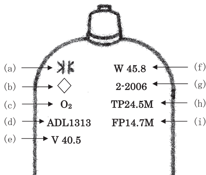
図 9.1 高压ガス容器の刻印[(a)～(i) : 9.3(1)参照]
