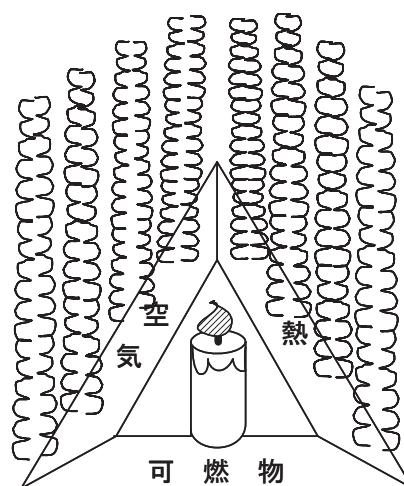
図 3.1 火の三角形
