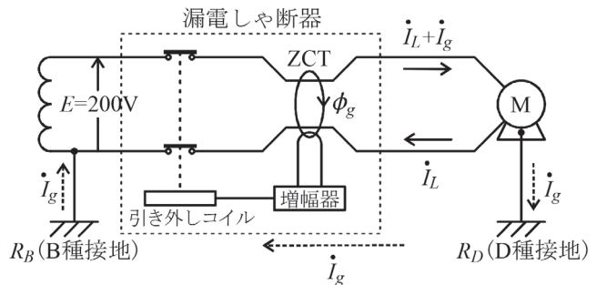
図 6.3 等価回路
