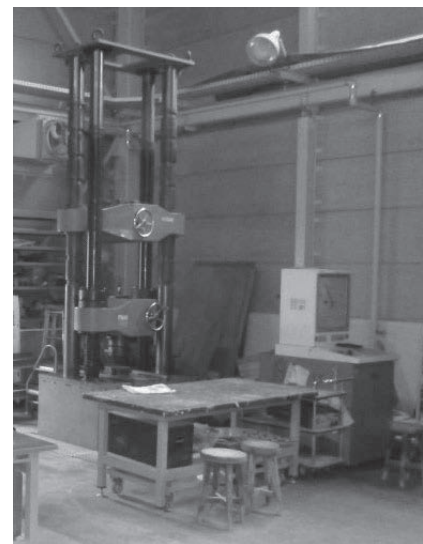
図 7.5 万能試験機
