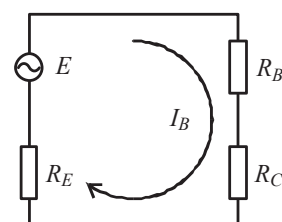
図 6.2 等価回路
