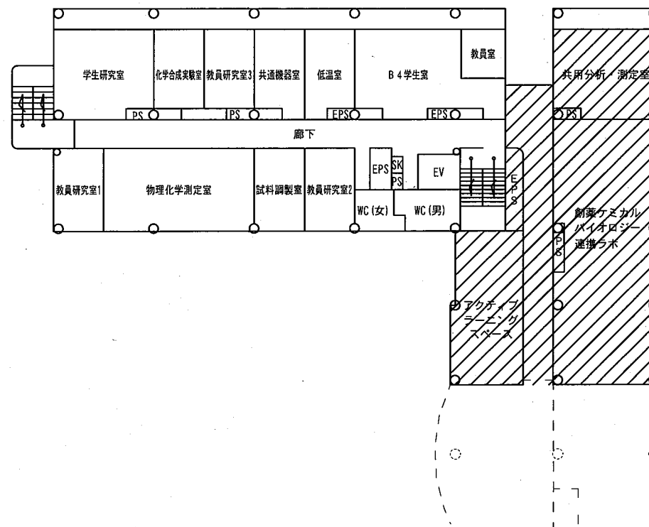
6 階平面図 (改修後)
