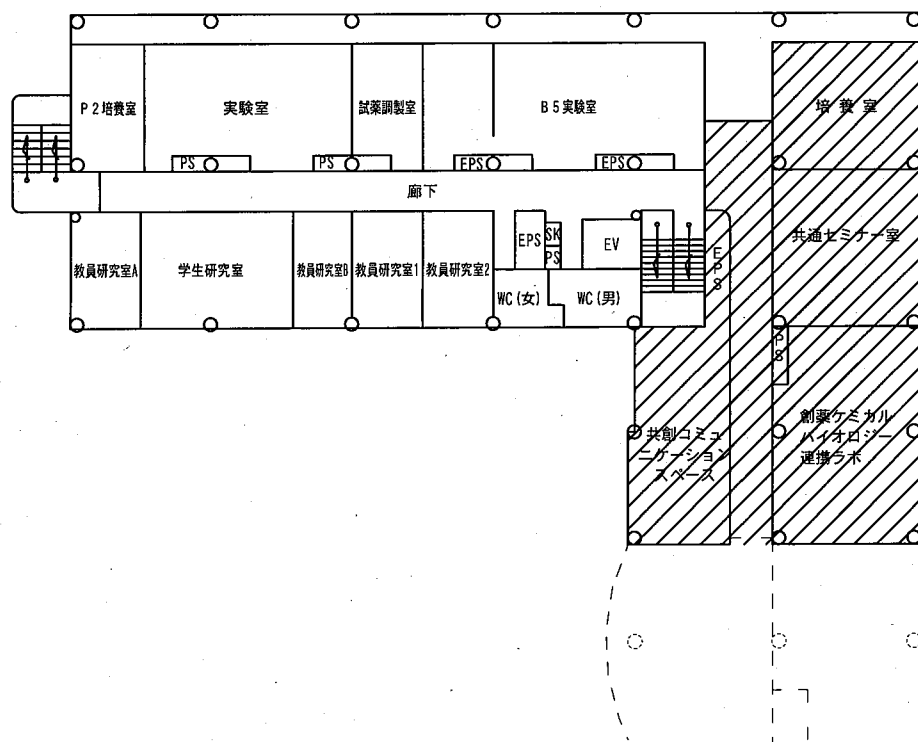
7 階平面図 (改修後)
