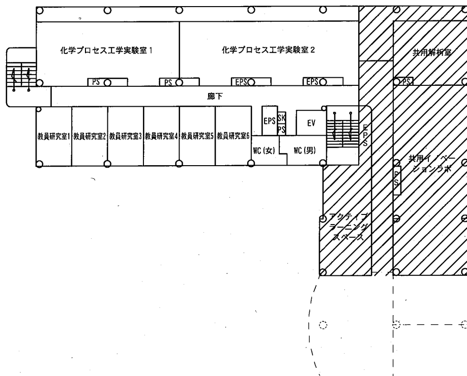
3 階平面図 (改修後)
