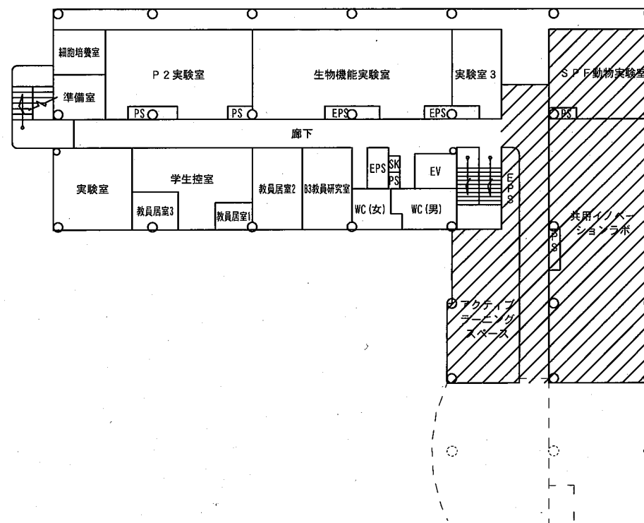
8 階平面図 (改修後)
