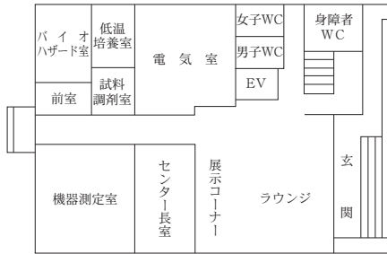
4 階平面図
