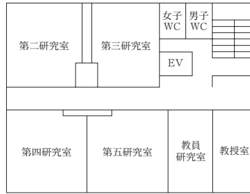
2 階平面図
