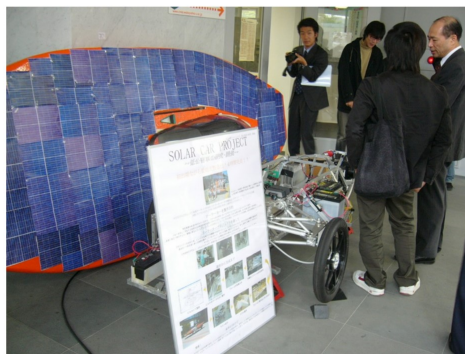
ソーラーカー（和太）
