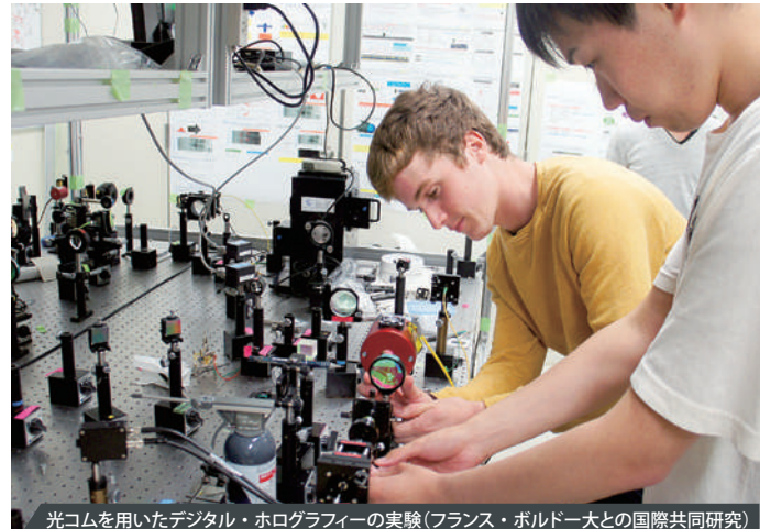
光コムを用いたデジタル・ホログラフィーの実験(フランス・ボルドー大との国際共同研究)
