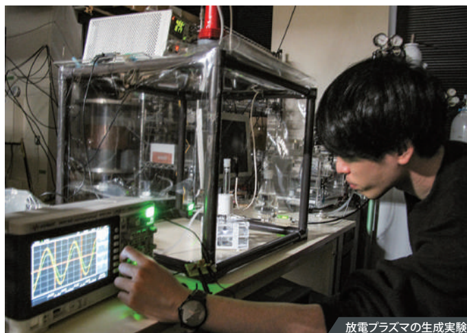
放電プラズマの生成実験
