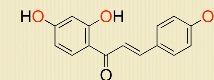
isoliquiritigenin
