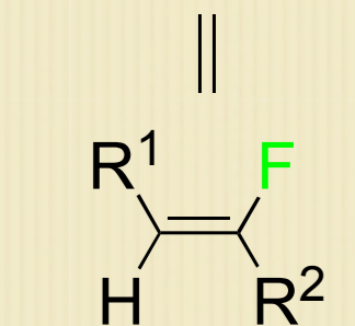
(Z)-fluoroolefin
