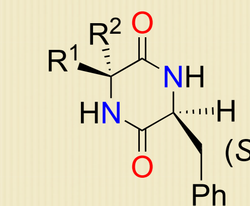
diketopiperazine
