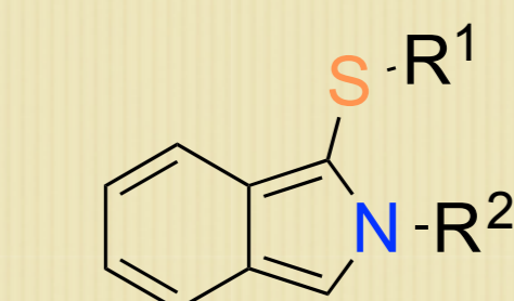
isoindole
