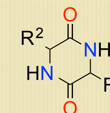
diketopiperazine
